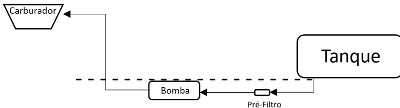
Esquema de instalação recomendado
