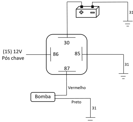
Esquema de instalação elétrica recomendada (relé não incluso)
